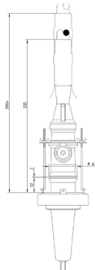
Cotes d'encombrement en mm
